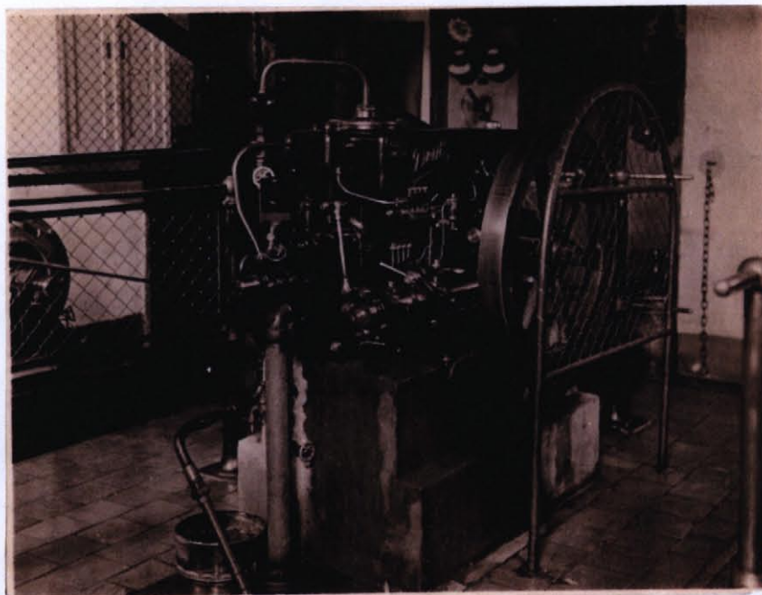
2) Karlovy Vary - Deuterův benzínový motor pro kompresory potrubní pošty
